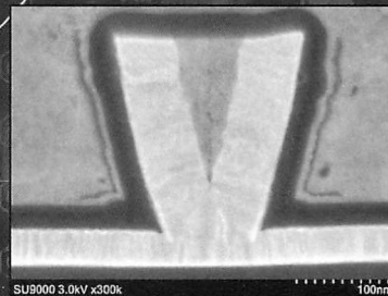
【試料】 ハードディスク ドライブヘッド
